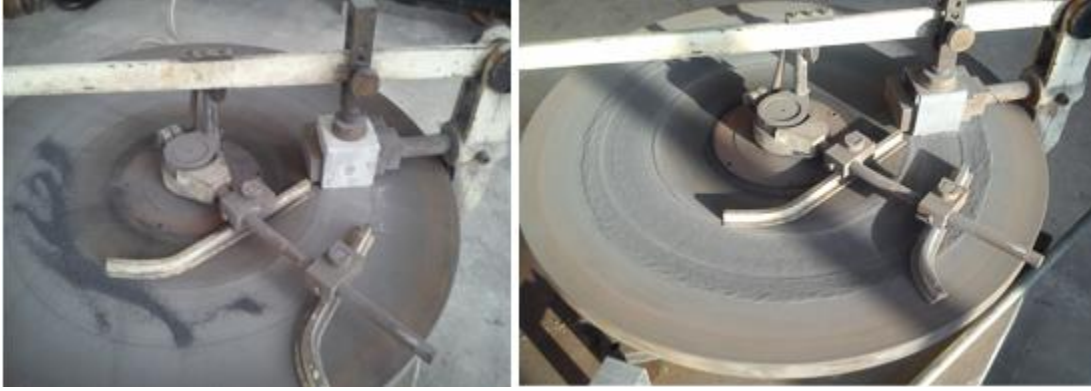
Şekil 6. Böhme Test Cihazı
