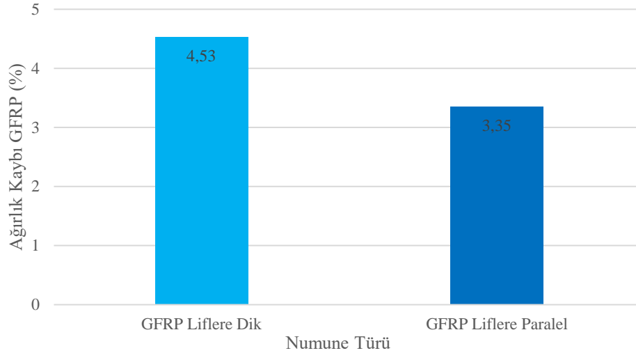
Şekil 9. GFRP Profil Ağırlık Kayıpları
