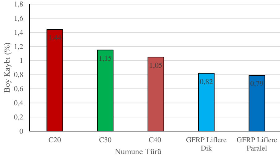
Şekil 7. Tüm Numuneler Boy Kayıpları
