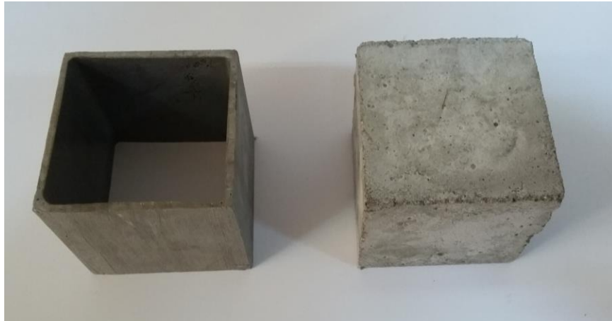
Şekil 5. GFRP Kutu Profil ve Beton Aşınma Numunesi
